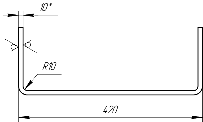
Дет. поз. 1 (1:5)
